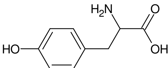
Tyrosine
