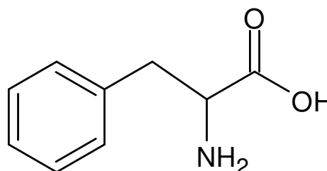
Phénylalanine
